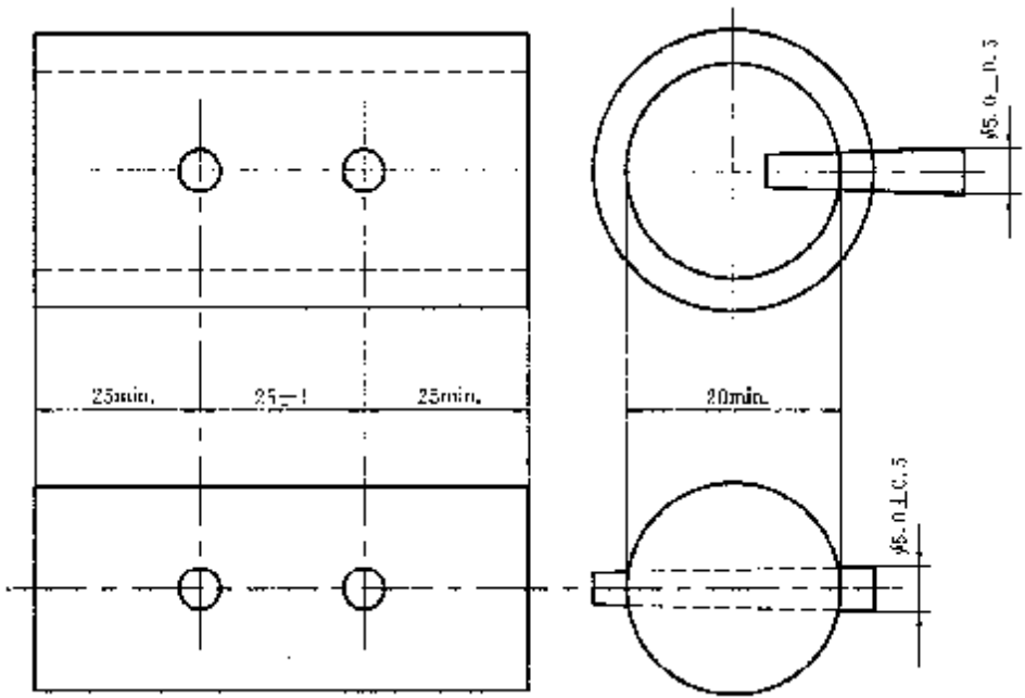
a) 带锥销电极的平板试样
