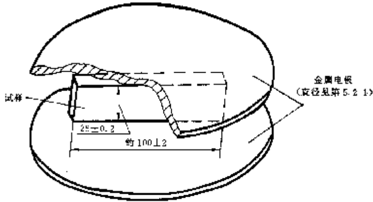
图 4 平行于表面(和沿层)试验用的电极装置
