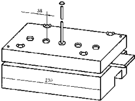
a) 装置的总装图
