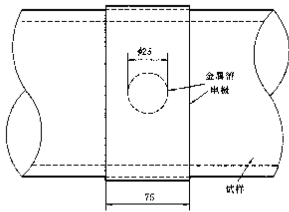
图 3 对内径大于 100 mm 的管子作垂直表面试验的电极装置
